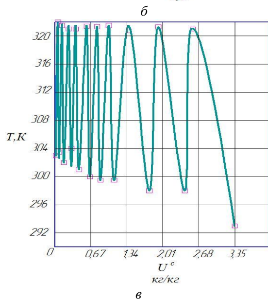
Рисунок 3 – Кривая сушки и скорости сушки груш (а) при ступенчатом режиме СВЧ - конвективной сушки груш, термограмма (б) и температурная кривая (в) при ступенчатом режиме СВЧ - конвективной сушки груш
